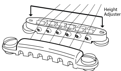
Höheneinstellschraube
