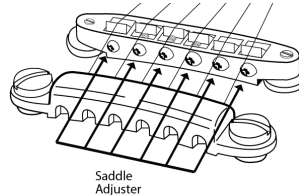
Intonatie instelschroef (voor elke snaar)
