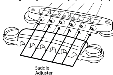
Źręba regulacji intonacji (dla każdej struny)
