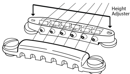
Höheneinstellschraube
