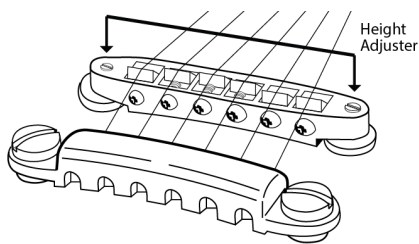
Śruba regulacji wysokości
