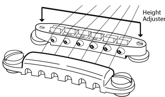
Hoogte instelschroef
