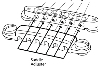
Intonationseinstellschraube (für jede Saite)
