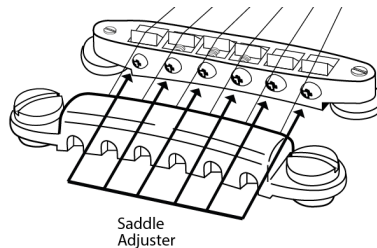
Śruba regulacji intonacji (dla każdej struny)
