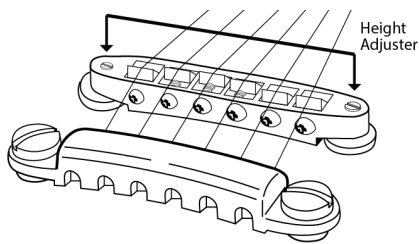
Vis de réglage de la hauteur
