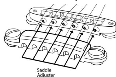
Intonatie instelschroef (voor elke snaar)
