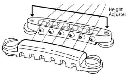
Hoogte instelschroef
